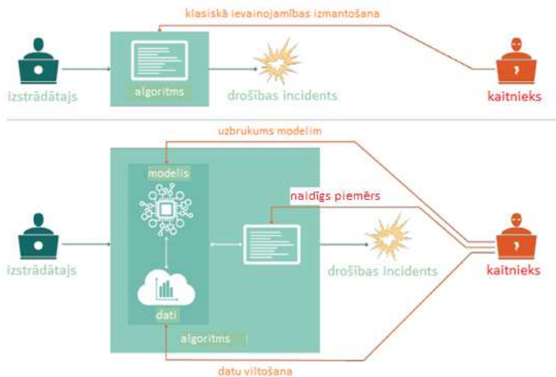
6.attēls. Uzbrukumu iespējas MI sistēmās 106 .
