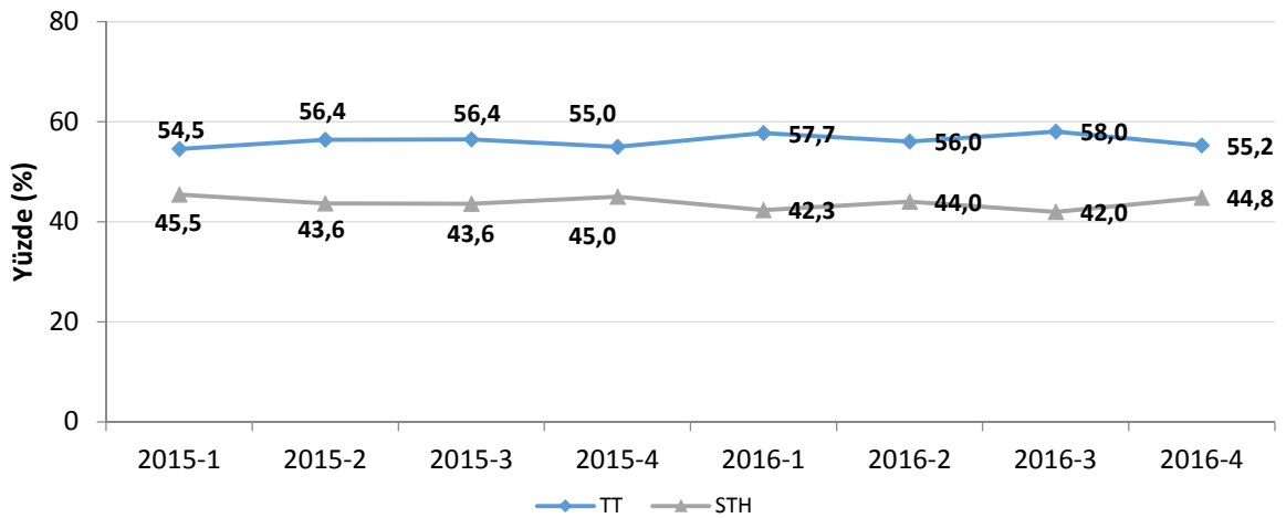
Şekil 2-9 STH–TT Çağrı Başlatma (Mobile doğru) Trafiki Kıyaslaması, %
