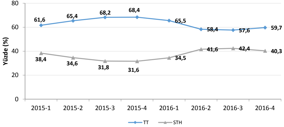
Şekil 2-10 STH–TT Çağrı Başlatma (Yurtdışına doğru) Trafiği Kıyaslaması, %
