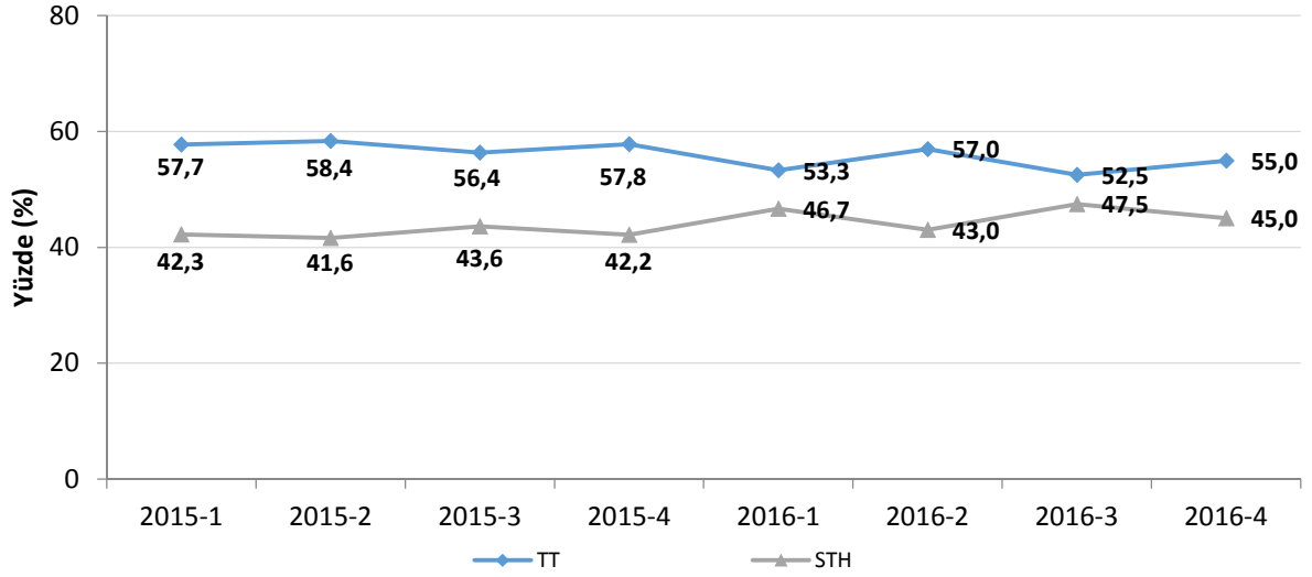
Şekil 2-8 STH–TT Çağrı Başlatma (Şehirlerarası) Trafiki Kıyaslaması, %
