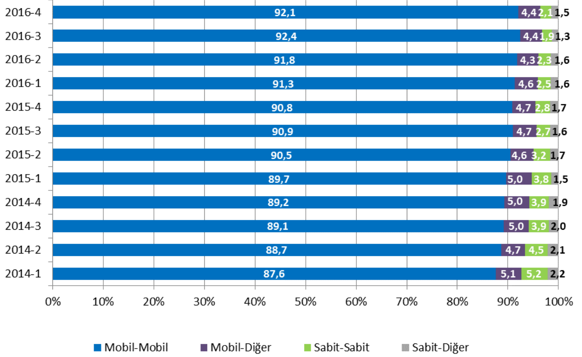
Şekil 1-6 Trafik Dağılımı, %
