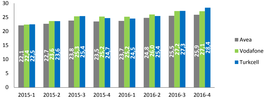
Şekil 4-29 Mobil ARPU, ₺
