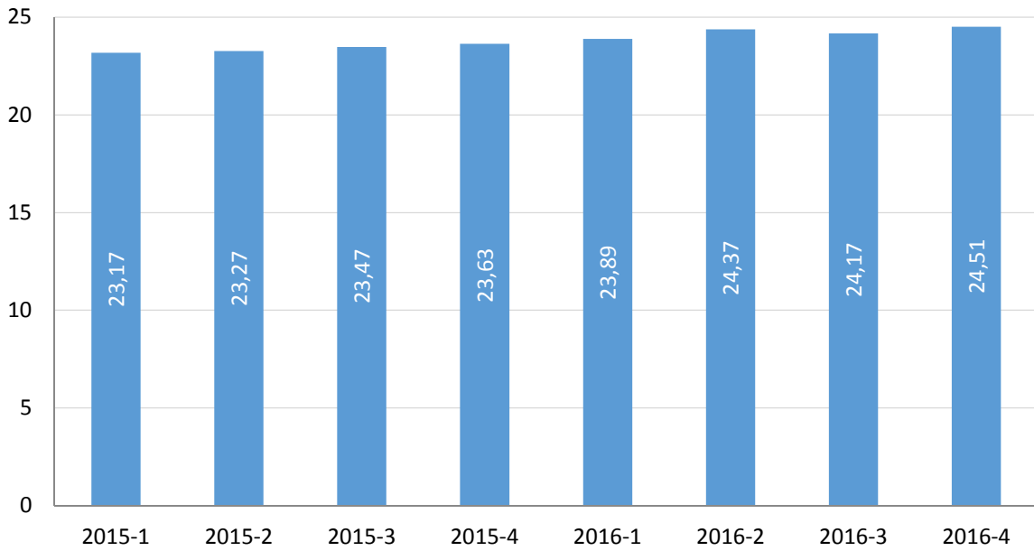
Şekil 2-16 Sabit ARPU, ₺
